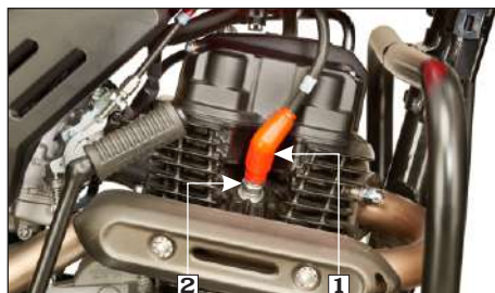
(1) Tapa supresor de ruido (2) Bujía
