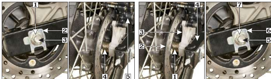
(1) Tuerca del eje trasero (2) Placa indicadora (3) Eje (4) Collar lateral (5) Conjunto de pinza
